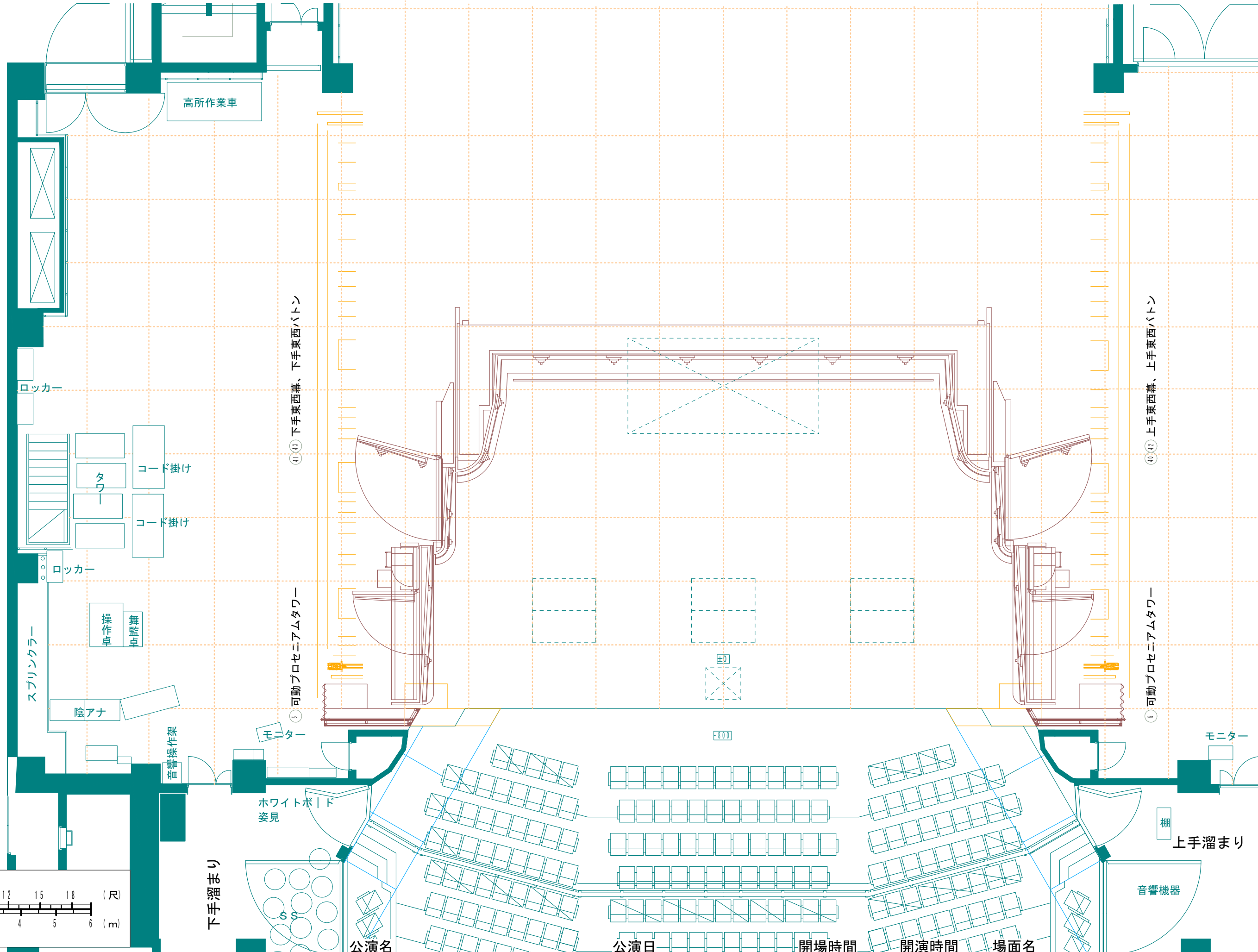
可児市文化創造センター主劇場GFL平面図 1/100 (A3)
