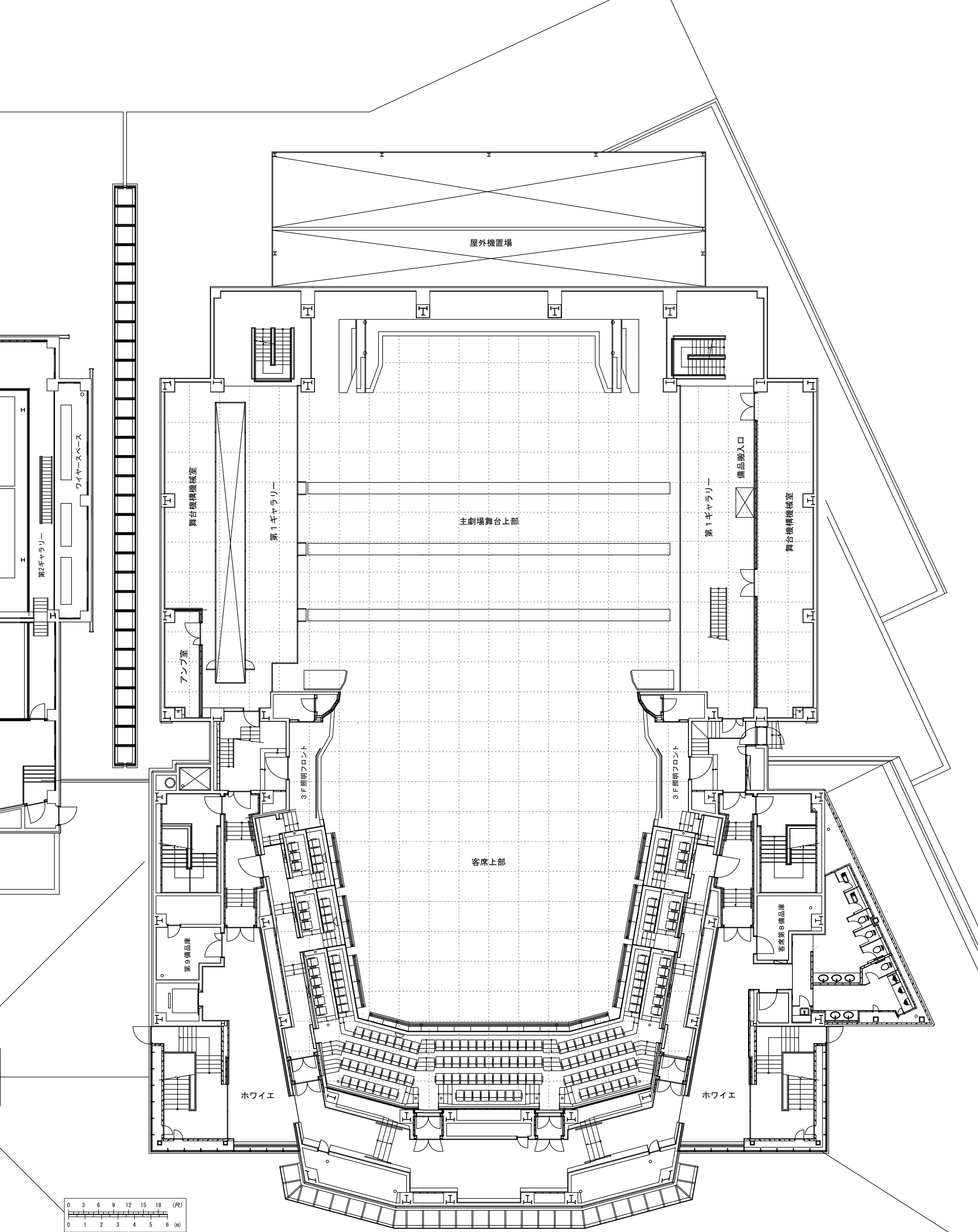
可児市文化創造センター 主劇場「宇宙のホール」 3F 平面図 1/200 (A3)
